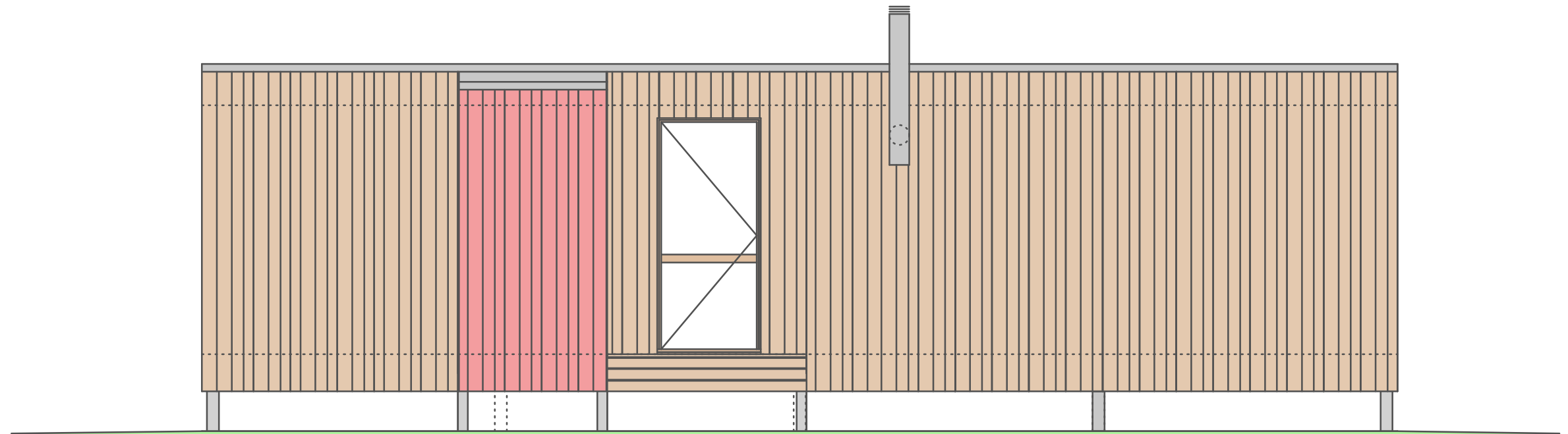
Ansicht Nord
